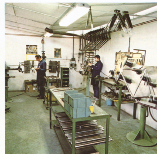
Reparto assemblaggio e saldatura Assembly and welding department Montageabteilung und schweisserei Atelier d'assemblage et soudage
