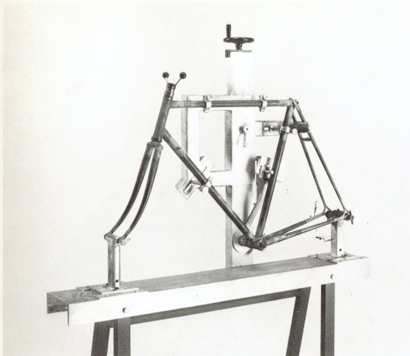
ART. 30 Maschera (DIMA) per costruire telai su misura
