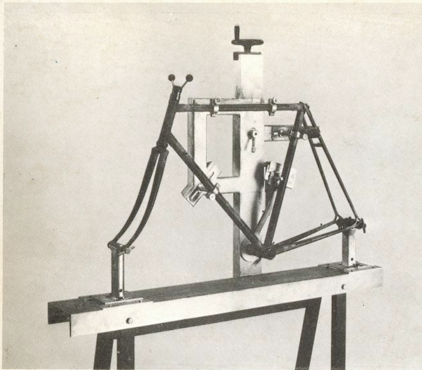
MASCHERA PER COSTRUZIONE TELAI SU MISURA
