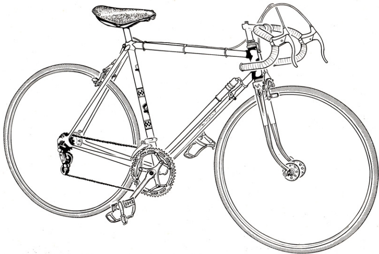
PA 10 - Caractéristiques : Tubes PEUGEOT, fourreaux de fourche chromés, jante MAVIC SPORT 700 C, moyeux AV et AR grands flasques, dérailleur AV et AR PRESTIGE, manivelle 3 branches, double plateau 46x50, freins MAFAC, RACER.
