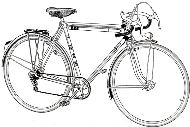
PL 8 - CARACTÉRISTIQUES : Roues de 700 C, jantes chromées, dérailleur AR PRESTIGE, freins MAFAC RACER, guidon, pédales et selle course, porte-bagages sport, garde-boue métal léger.
