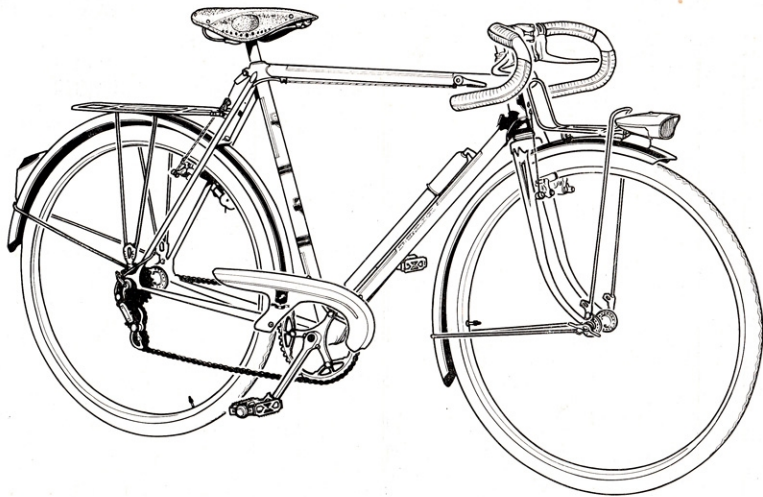
H 50 - CARACTÉRISTIQUES : Roues de 650, jantes chromées, freins à tirage central Cantilever BEBO, pare-chaîne acier, garde-boue métal léger, guidon randonneur, porte-bagages AV et AR, dérailleur AR.
