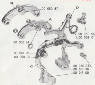
Pour roues de 26x1,75 (PLE) For 26x1,75 wheels (PLE) Für 26x1,75 Räder (PLE) Pour roues de 20x1,75 (DA-PA) For 20x1,75 wheels (DA-PA) Für 20x1,75 Räder (DA-PA) A=00 051 53 C=00 051 73 B=00 051 54 D=00 051 72
