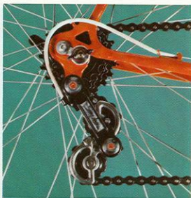
Rear derailleur Simplex Criterium.
